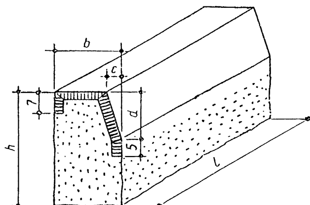
Rys. 2. Krawężnik rodzaju B
